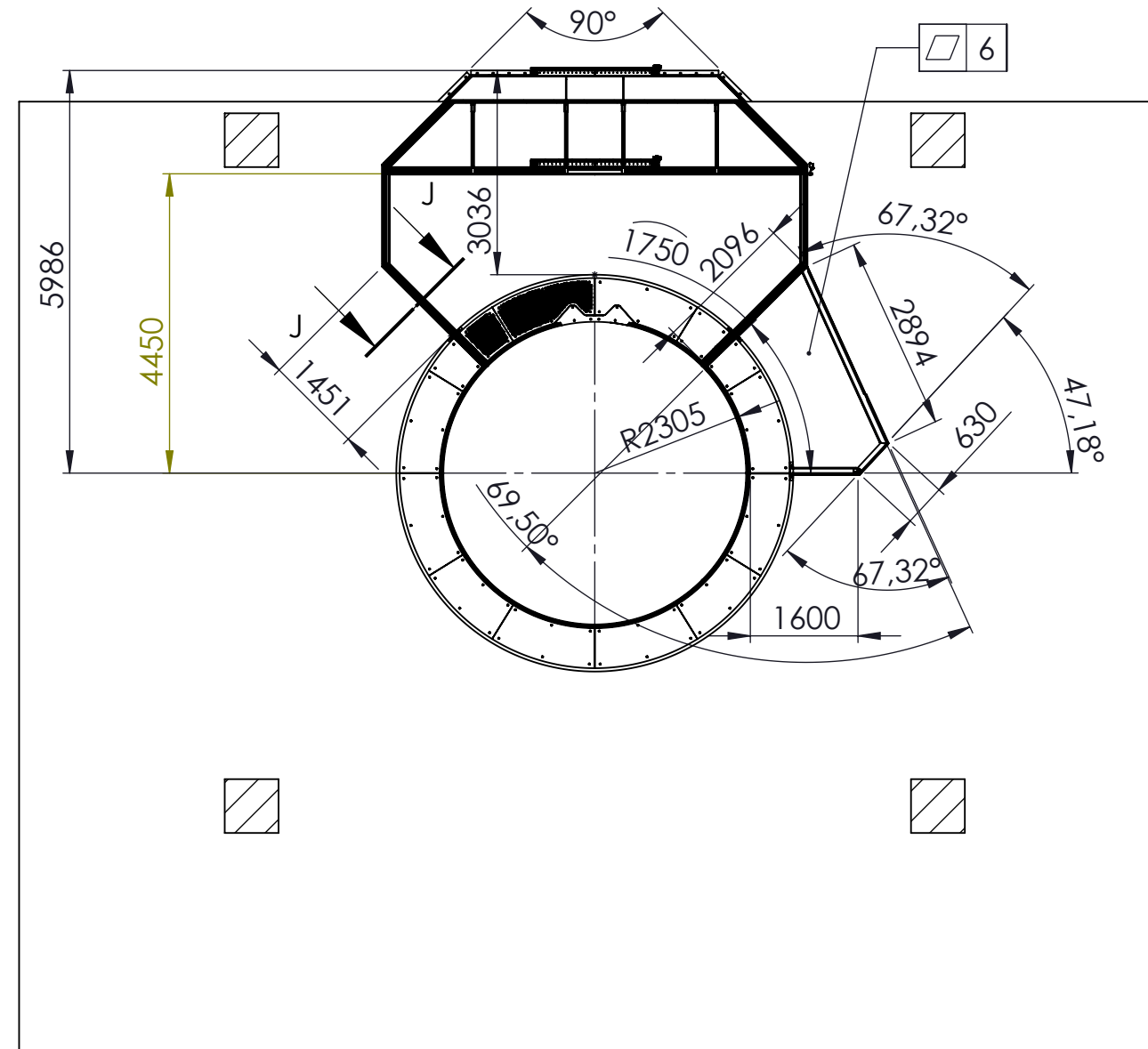
F-F (1 : 100)
