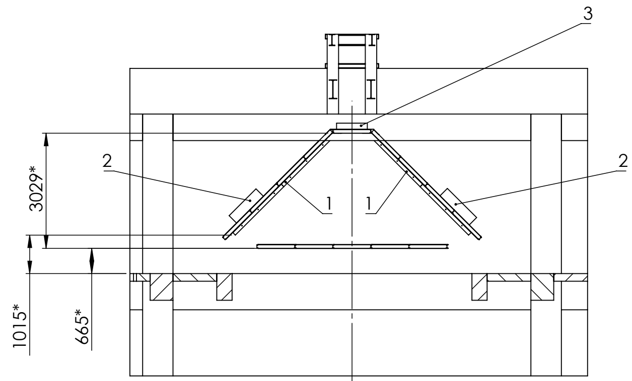
D-D (1 : 100)
