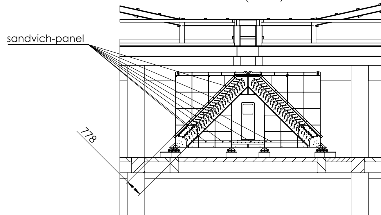
C-C (1 : 100)
